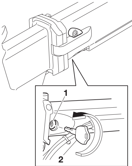
1 フレームロックレバー
