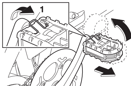
1 ペダル折畳レバー
