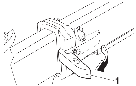
1 フレームロックレバー
