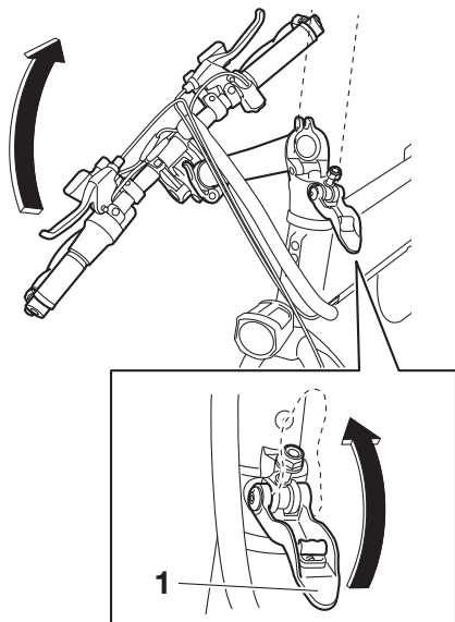
1 ハンドル折畳レバー
